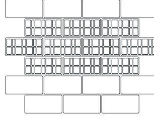
Combinación con ladrillo trabado
