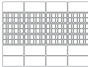
Combinación con ladrillo sin traba
