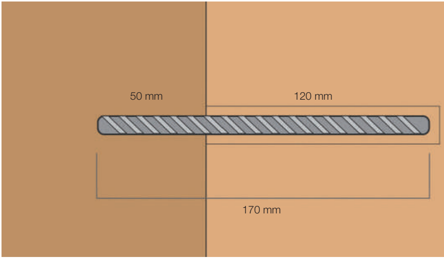
Medidas de anclajes
