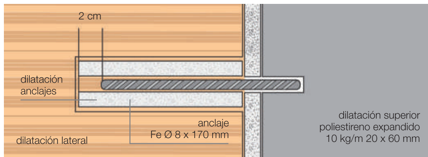
Medidas de la manga de poliestireno
