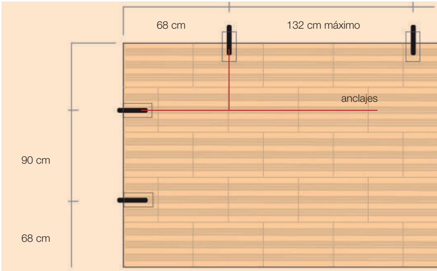
Separaciones entre anclajes
