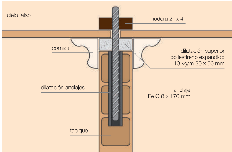
Refuerzo para cielo entramado
